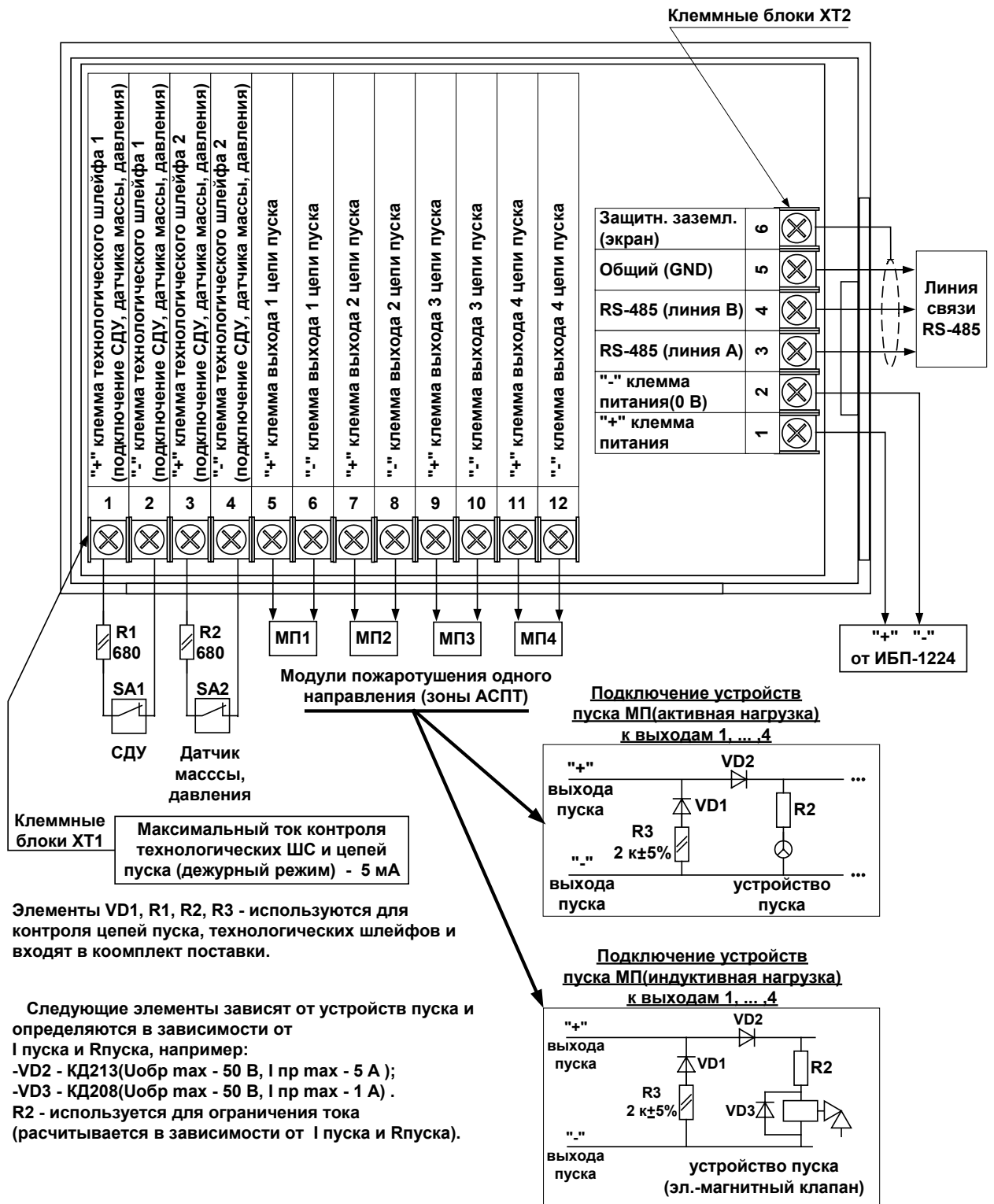
Рис. 5 Схема подключения СКУП
