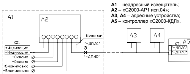
Рисунок 1 Схема соединений
