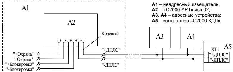
Рисунок 1 Схема соединений
