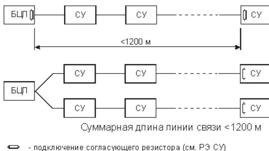
Рис. 1 Варианты включения СУ в линию связи
