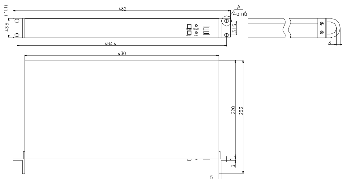
Рис. 9 Исполнение 2 - габаритные и присоединительные размеры
