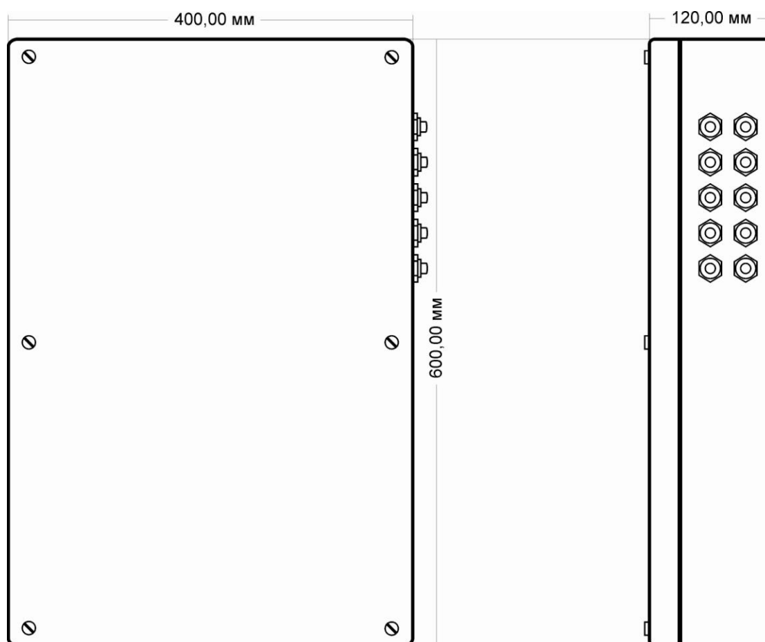
Исполнение 5 - габаритные и присоединительные размеры
