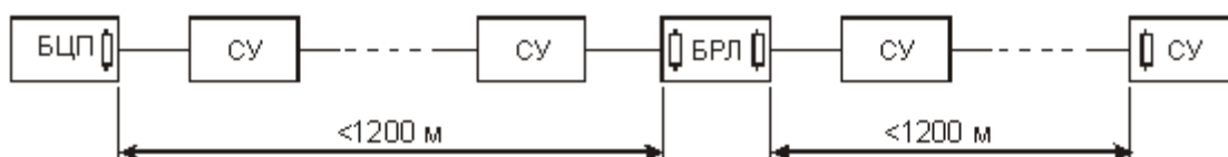
Рис. 2 Использование БРЛ-03 для удлинения линии связи
