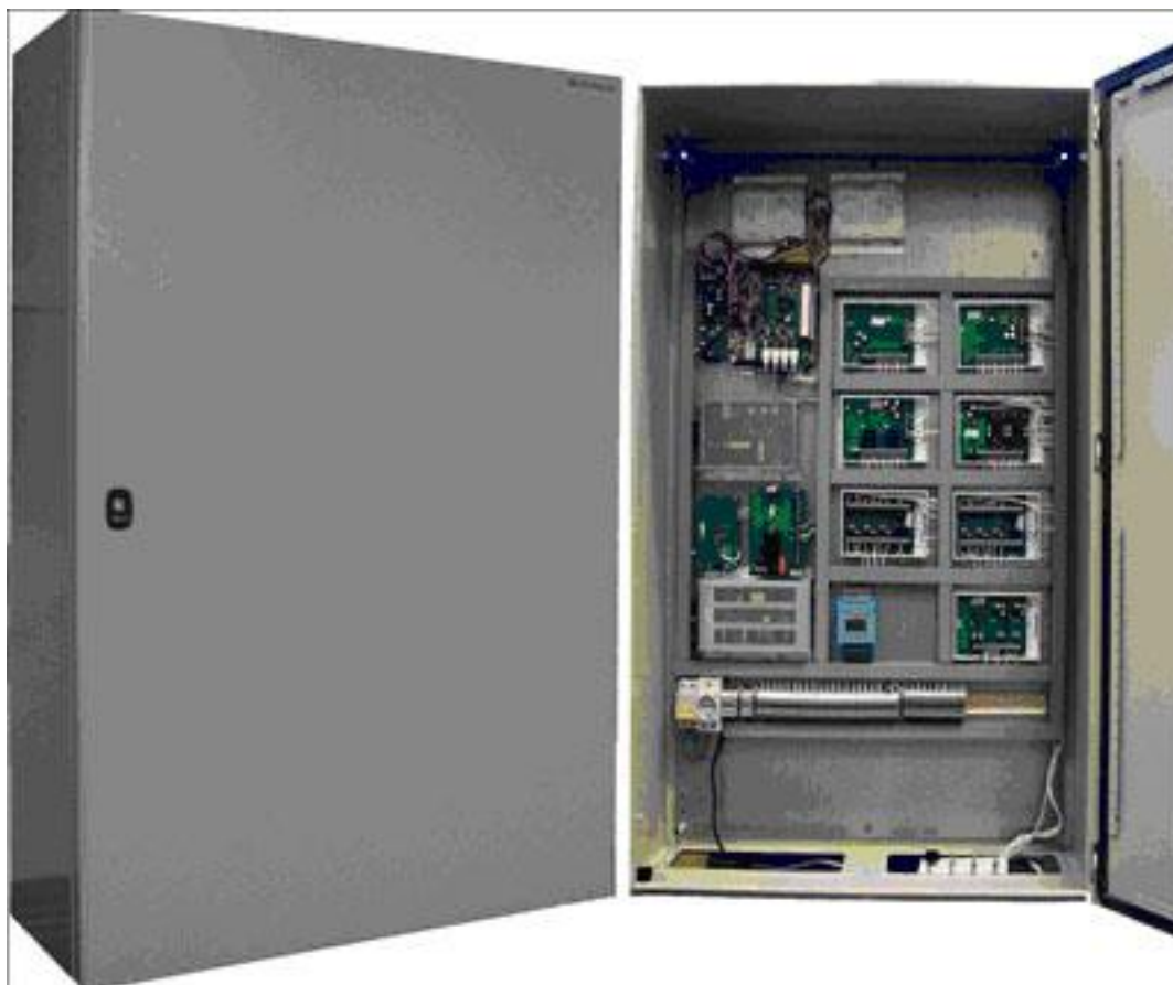
Исполнение 3 - внешний вид
