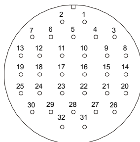
Рис. 9 Разъем для подключения БР
