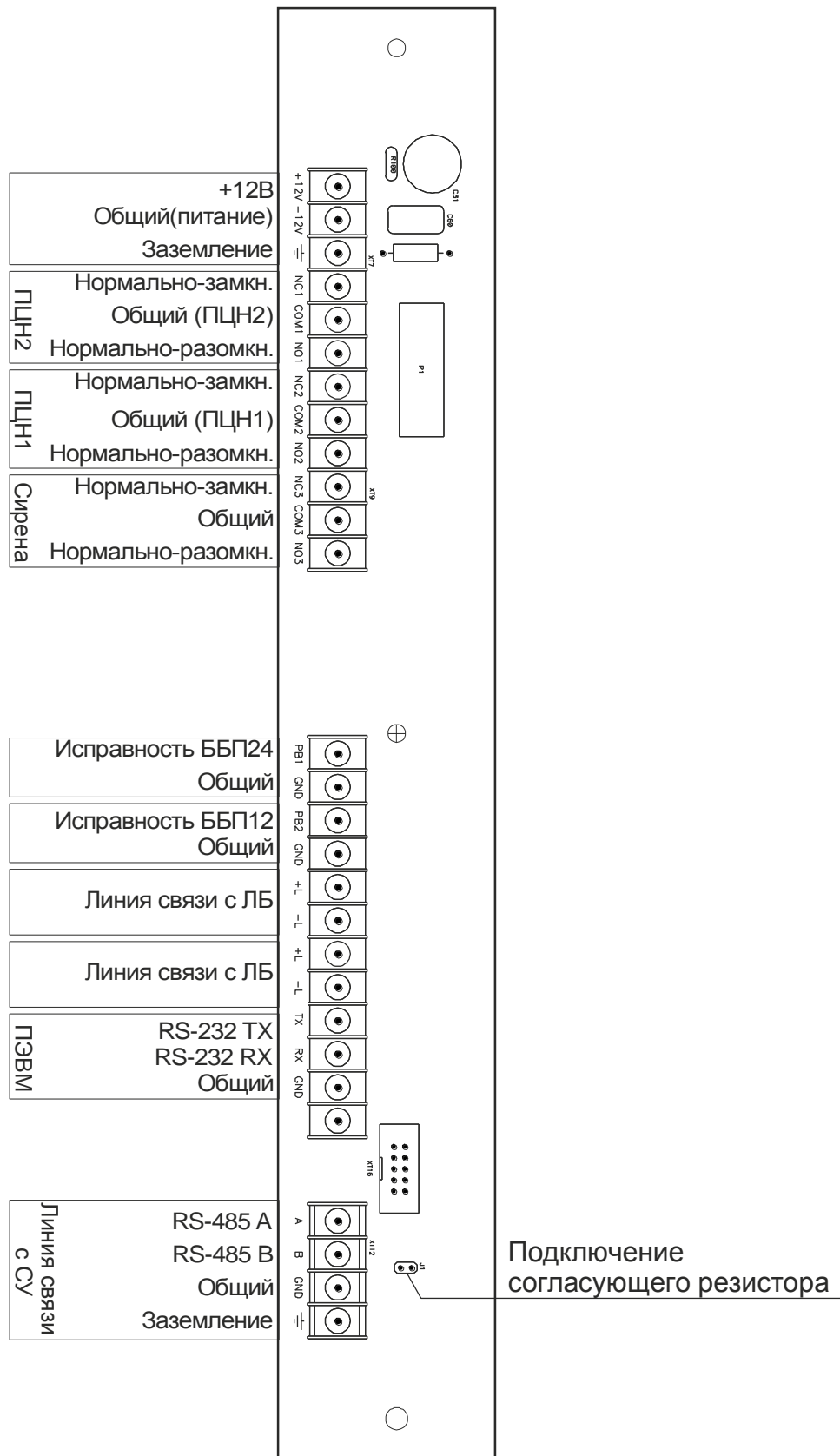
Рис. 8 Схема подключения БЦП
