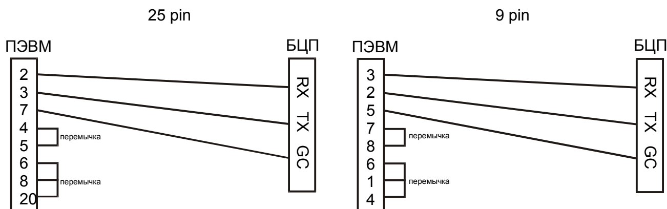
Рис. 10 Схема распиновки кабеля для подключения ПЭВМ
