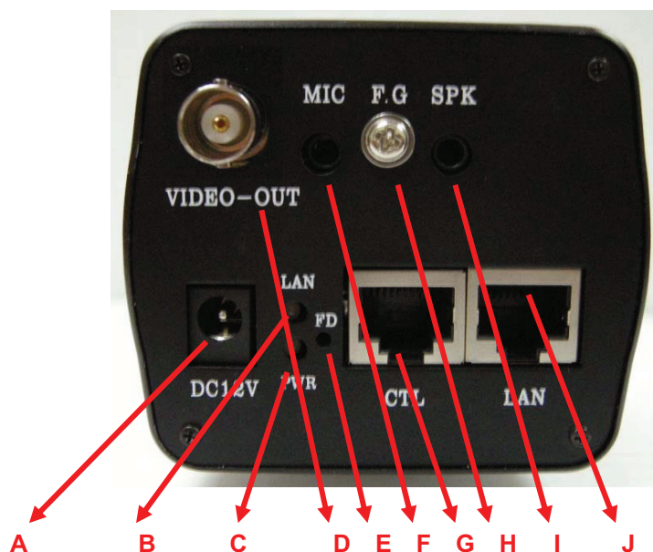
Рисунок 3. Вид сзади MDC-i4220CDN, MDC-i4220TDN
